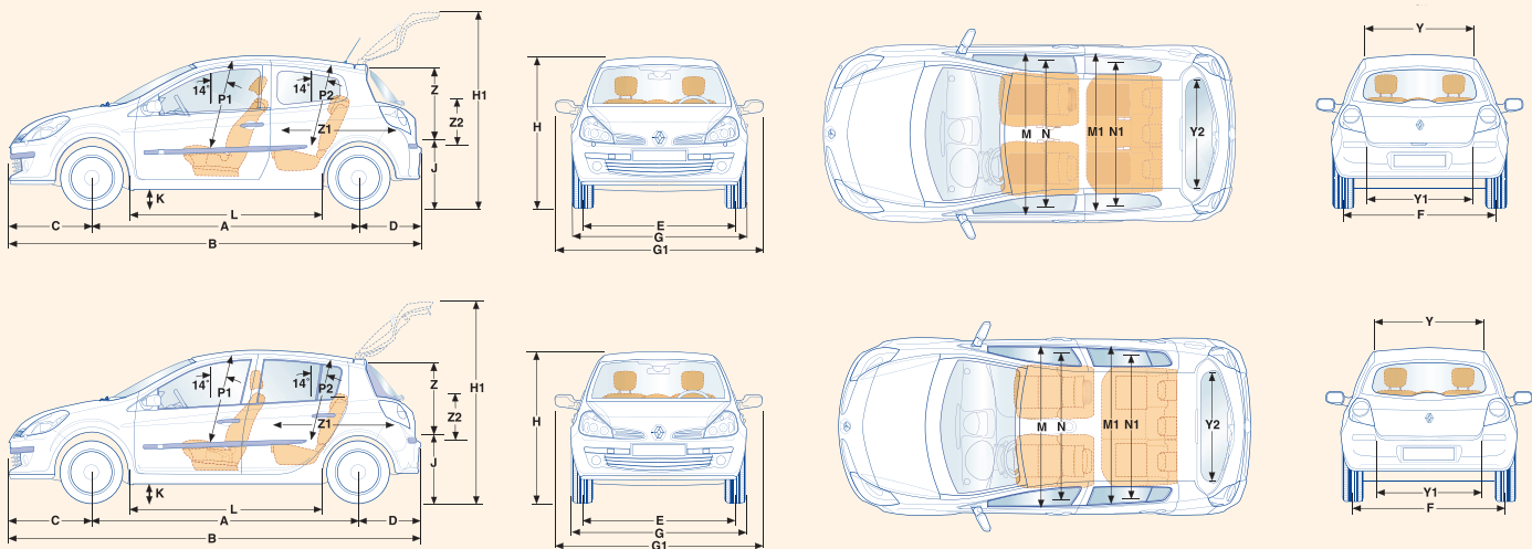
Plan côté (mm)
